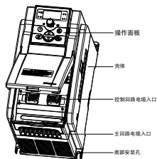
图 1-3 III类变频器外观及部件名称
