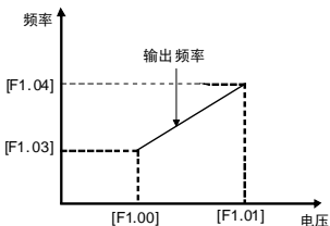
图 6-6 模拟输入量与设定频率对应关系图示
