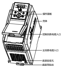
图 1-2 II类变频器外观及部件名称
